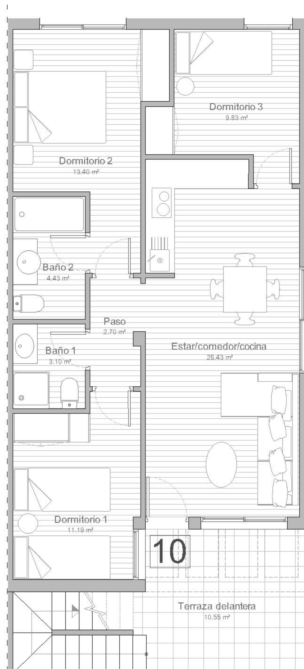
Planta primera
