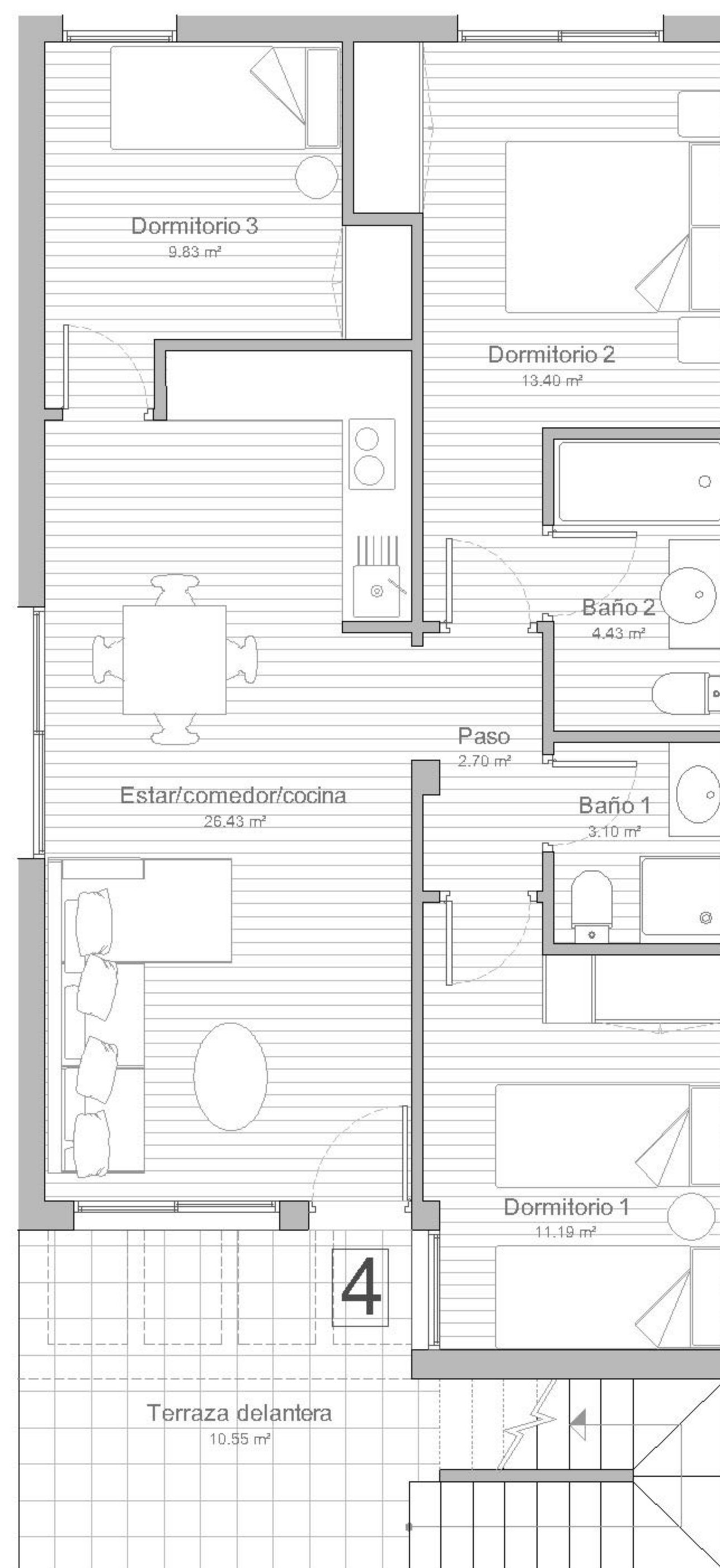
Planta primera
