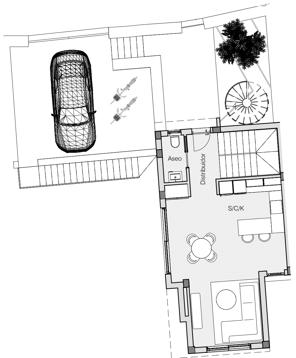
PLANTA BAJA
