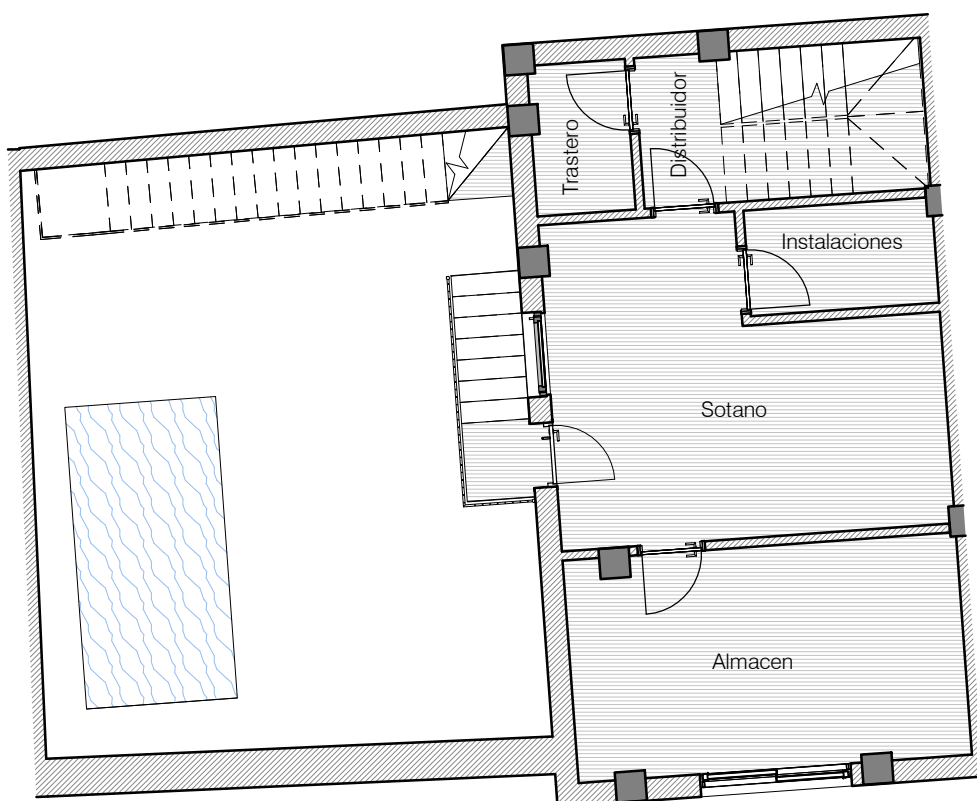
PLANTA SEMI-SÓTANO
