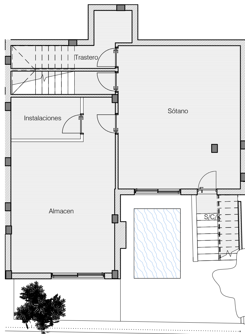
PLANTA SEMI-SÓTANO
