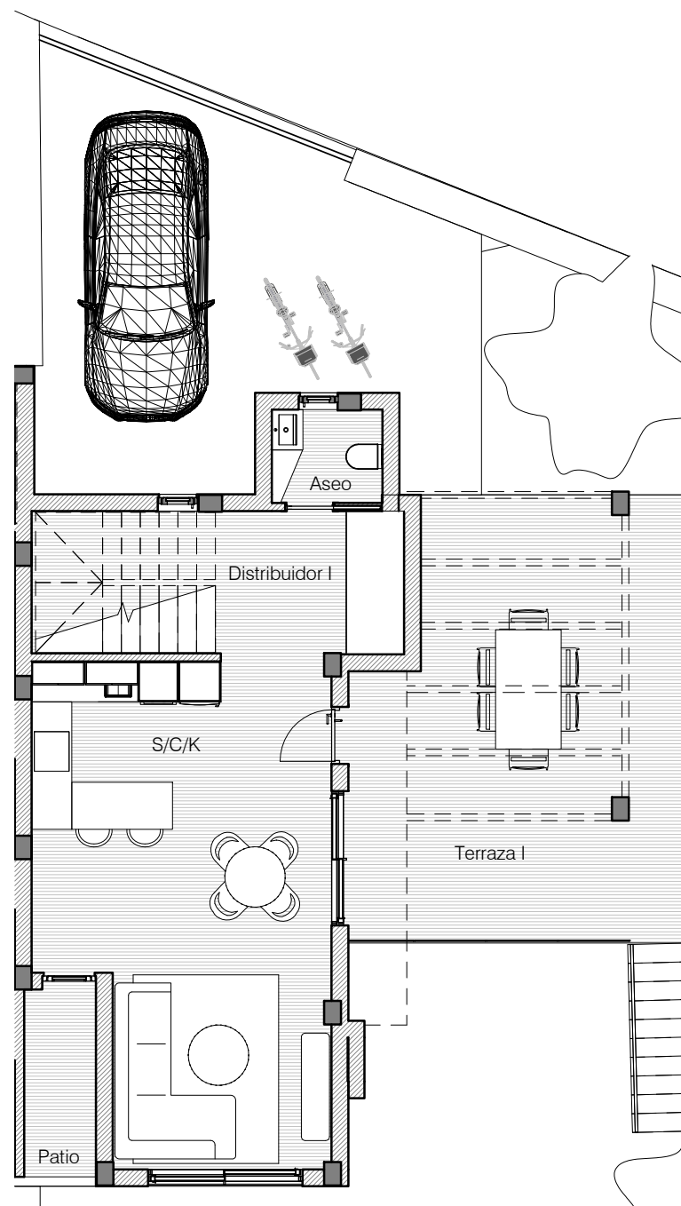
PLANTA BAJA
